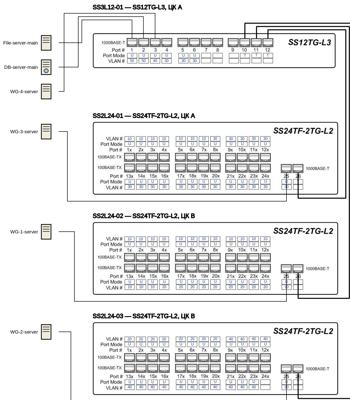
Рис. 4. Структура ЛВС с VLAN на интеллектуальных коммутаторах
